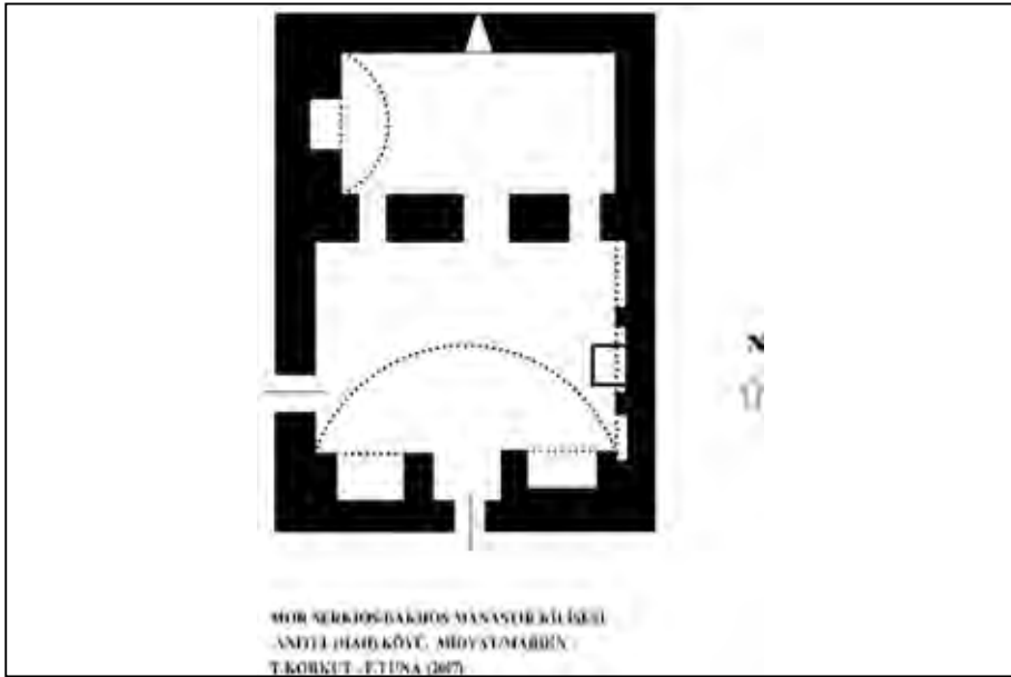
Plan 3: Anıtlı (Hah) Köyü, Mor Serkis Mor Bakos Manastırı Röleve Planı.
