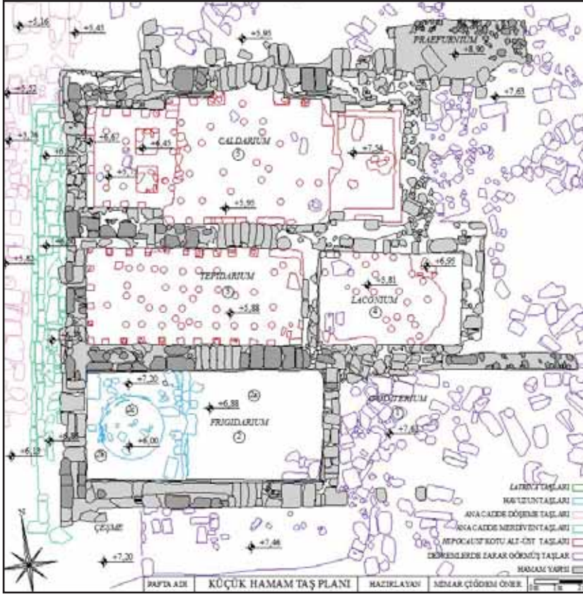
Resim 10: Phaselis Küçük Hamam taş planı (Ç. Öner).
