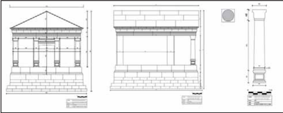
Resim 13: Tapınak planlı mezar, mevcut kalıntılar ışığında gerçekleştirilen restitüsyon önerisi (B. Gürel – M. Şimşek).
