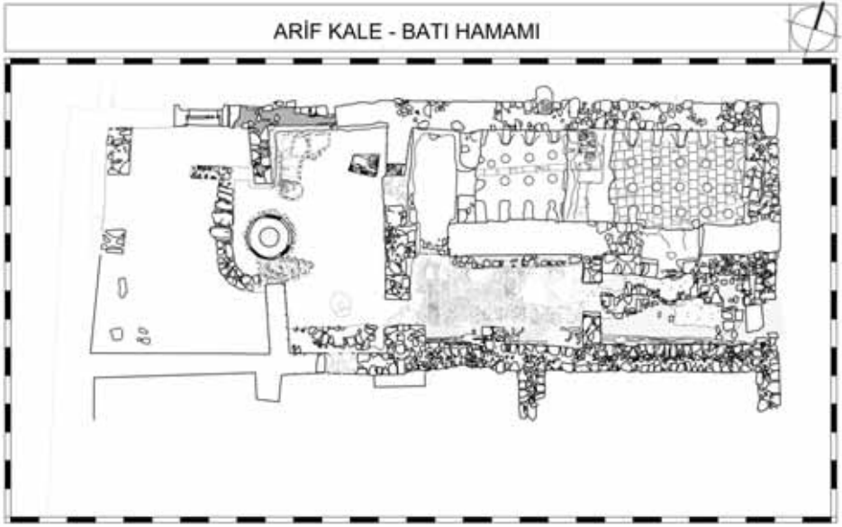
Plan 4: Arif Kale, Batı Hamam planı (2018).
