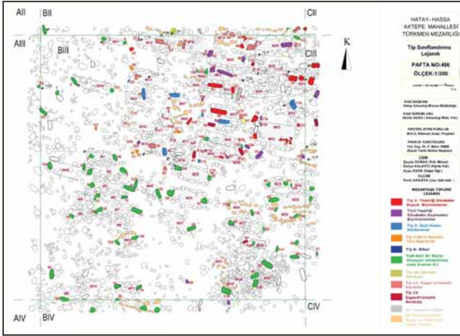
Çizim 2: B- III Açması vaziyet planı.
