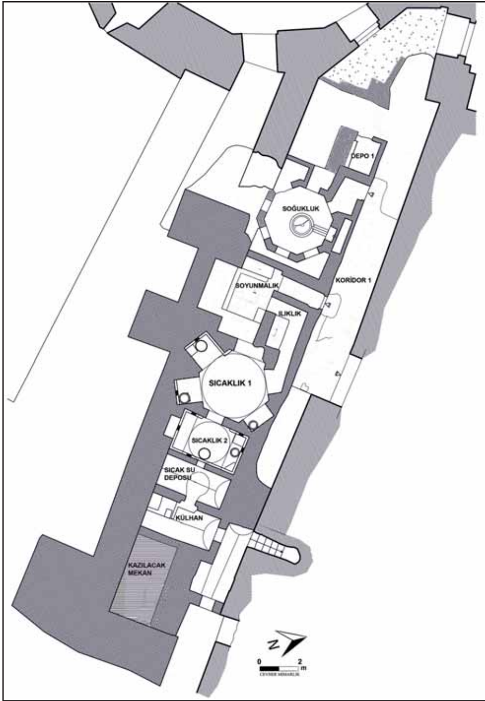
Plan 1: Saray Hamamı.
