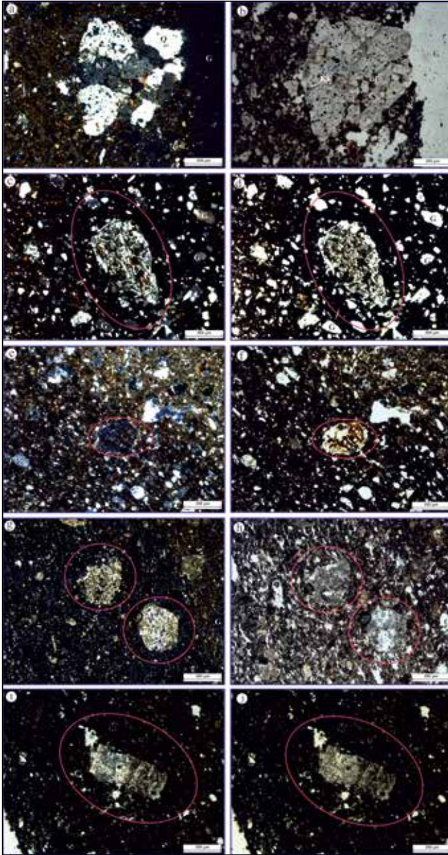
Şekil 5. Domuztepe çanak-çömlleklerinde gözlenen granitoyid (a: Çift Nikol b: Tek Nikol), bazalt (c: Çift Nikol d: Tek Nikol), Serpantinit (e: Çift Nikol f: Tek Nikol), Kireç taşı (g: Çift Nikol h: Tek Nikol) ve Mermer (ı: Çift Nikol j: Tek Nikol) görüntüleri (Q: kuvars, Bi: Biyotit, KF: K'lu Feldispat).
