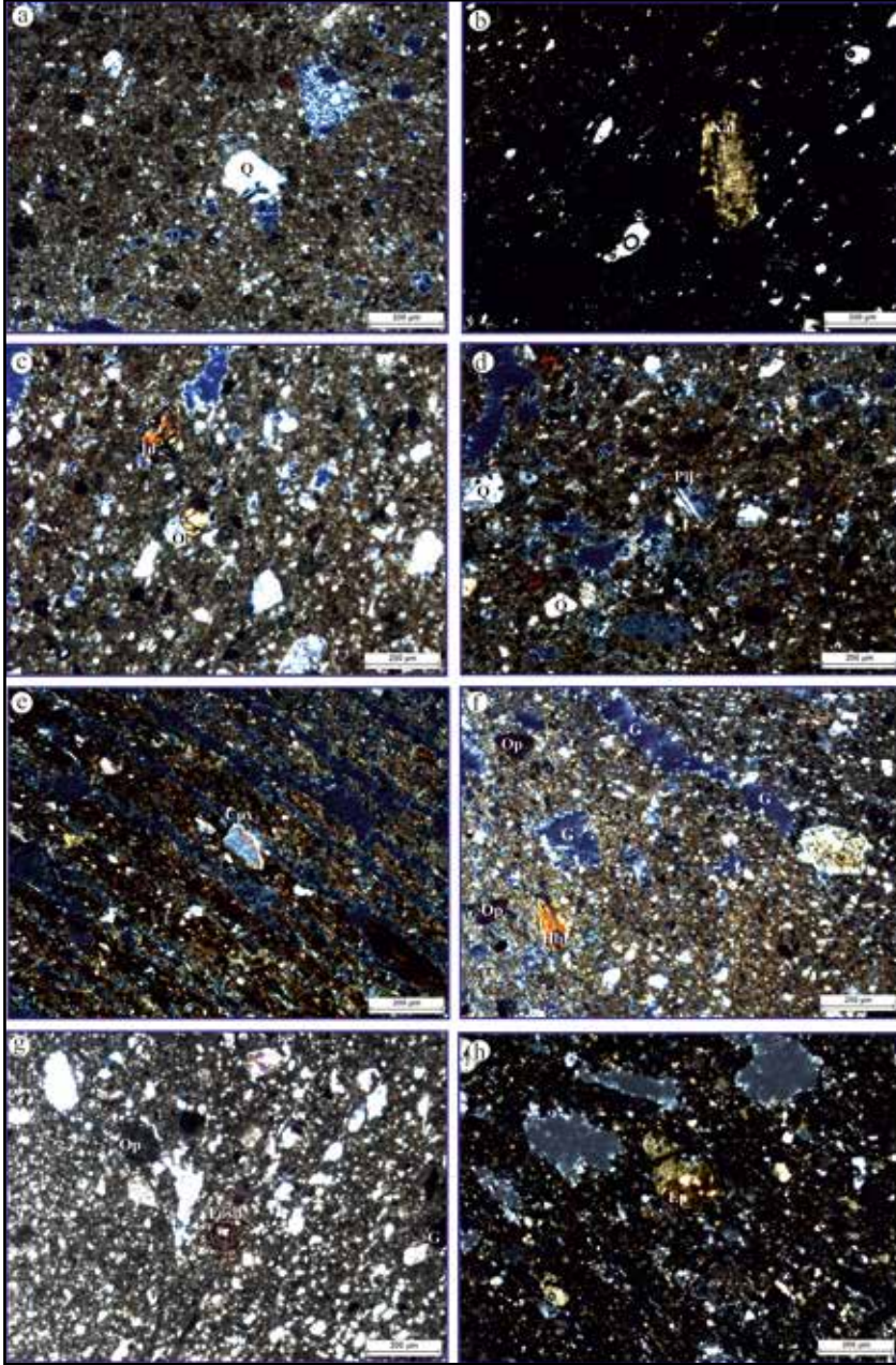
Şekil 4. Domuztepe çanak-çömlerinde tespit edilen mineraller ve fosil kalıntılarının çift nikol görüntüleri (Hbl: Hornblend, Plj: Plajiyoklas, Cpx: Klinopiroksen, Ol: Olivin, İd: İddingsit, Q: kuvars, Ep: Epidot, Kal: Kalsit, Op: Opak mineral)
