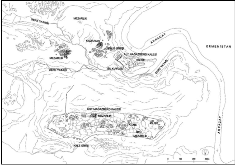
Çizim 2: Mağazberd Kalesi vaziyet planı (Çizen: A. Fenerci).
