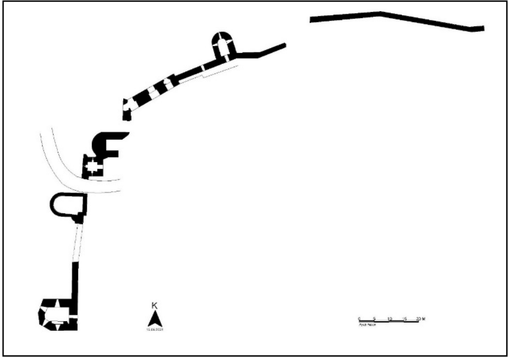
Çizim-2. Ayas Kalesi (Karadaki) planı
