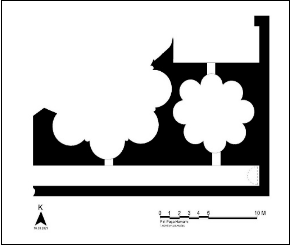
Çizim- 5. Piri Paşa Hamamı planı
