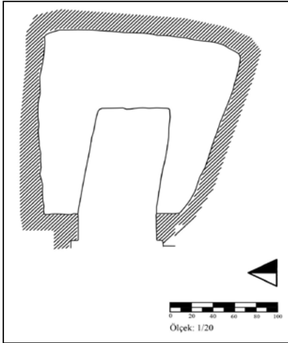
Resim 4: Çakırçal Köyü, Kaya Mezarı plan çizimi
