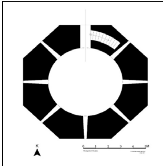
Çizim-3. Süleyman Kulesi planı
