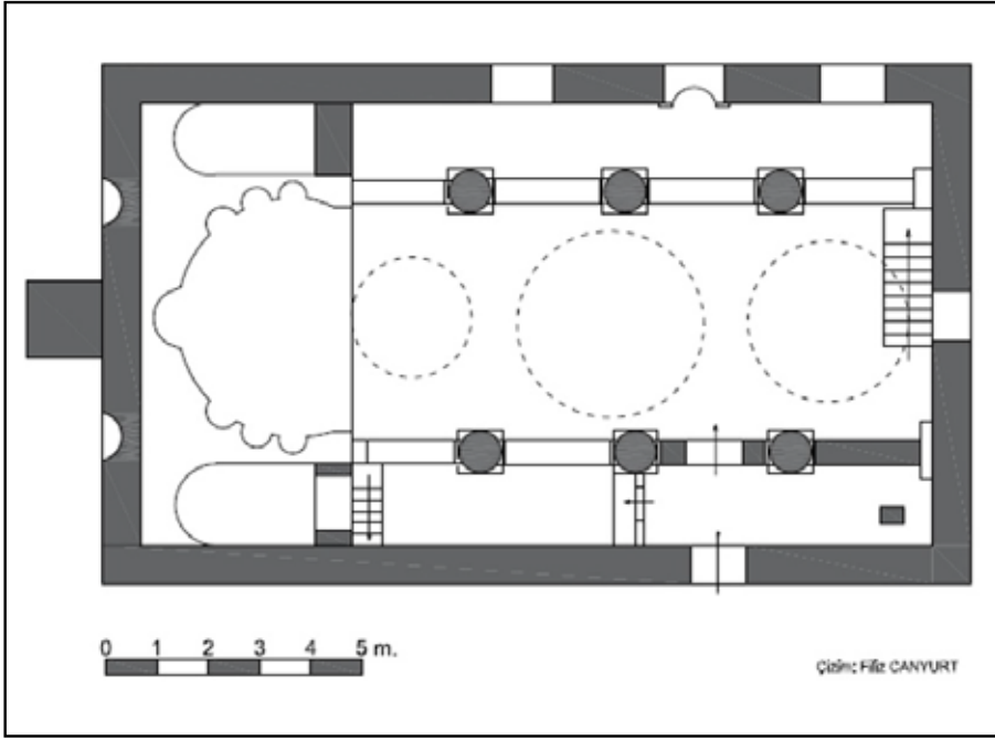
Çizim 4: Gölbelen Köyü Camii Rölövesi.
